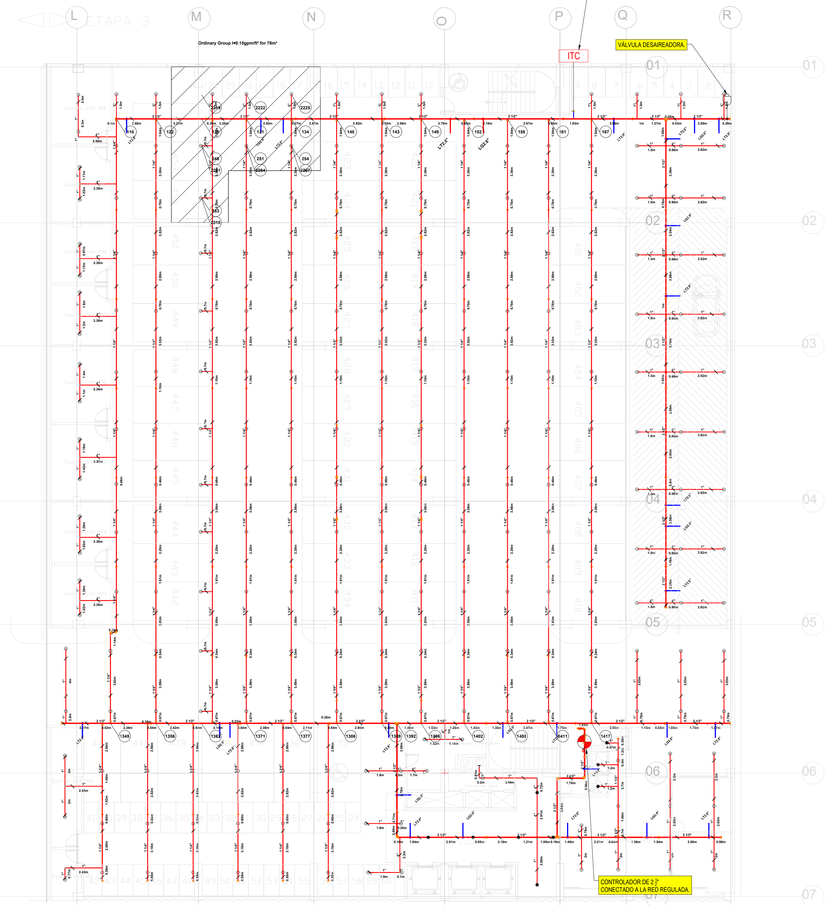
1 VISTA EN PLANTA EXTINCIÓN PISO 4 ESCALA 1:150
